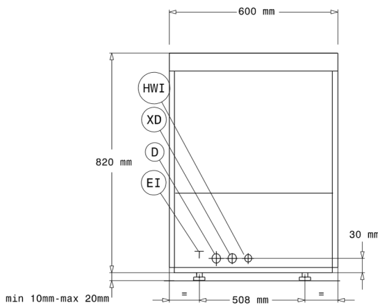
Zij aanzicht
